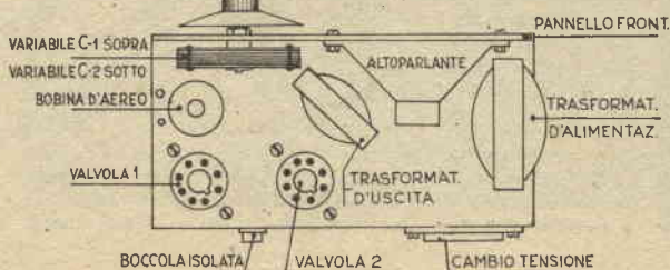
FIG.5 TELAIO PRONTO PER IL MONTAGGIO
