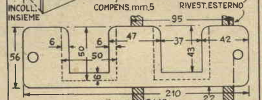
FIG. 7 TELAIO PORTAFOTO
