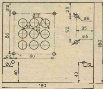
FIG.7 PANNELLO FRONTALE
